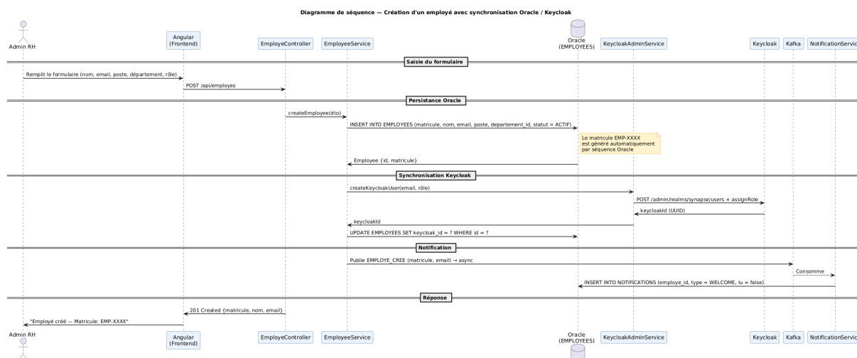
FIGURE 3.7 Diagramme de séquence : création d'un employé avec synchronisation Oracle–Keycloak
