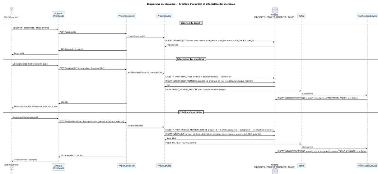
FIGURE 5.2 Diagramme de séquence : création d'un projet et affectation des membres
